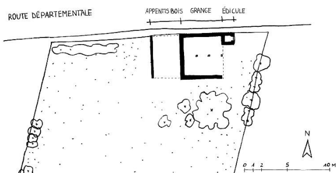
Figure 11 Avant réhabilitation de la grange
