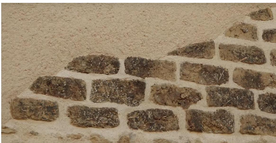
Figure 15 Façade nord partiellement enduite à la terre crue
