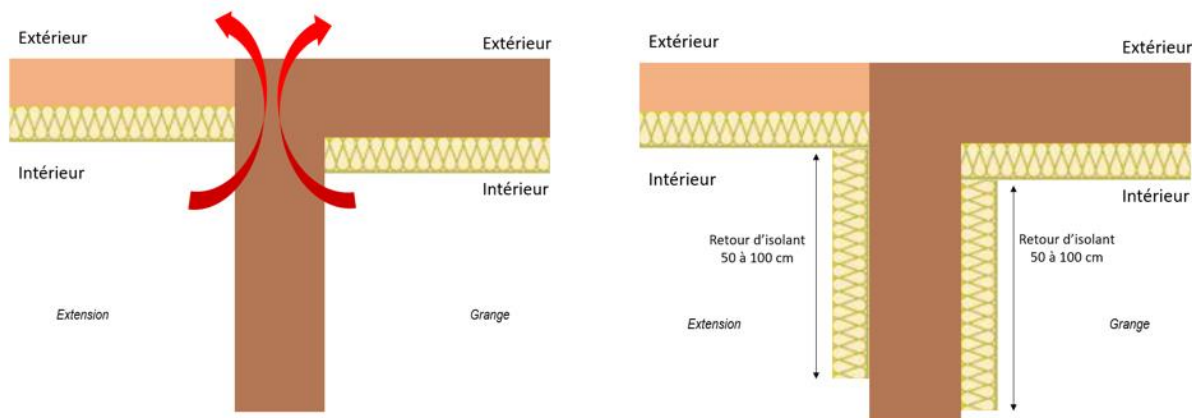
Figure 21 Avant et après traitement du pont thermique
